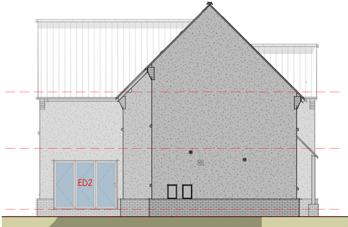
Elevation 04 - Left 1 : 100
