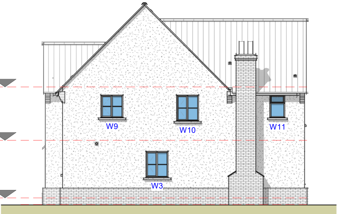
Elevation 02 - Right 1 : 100
