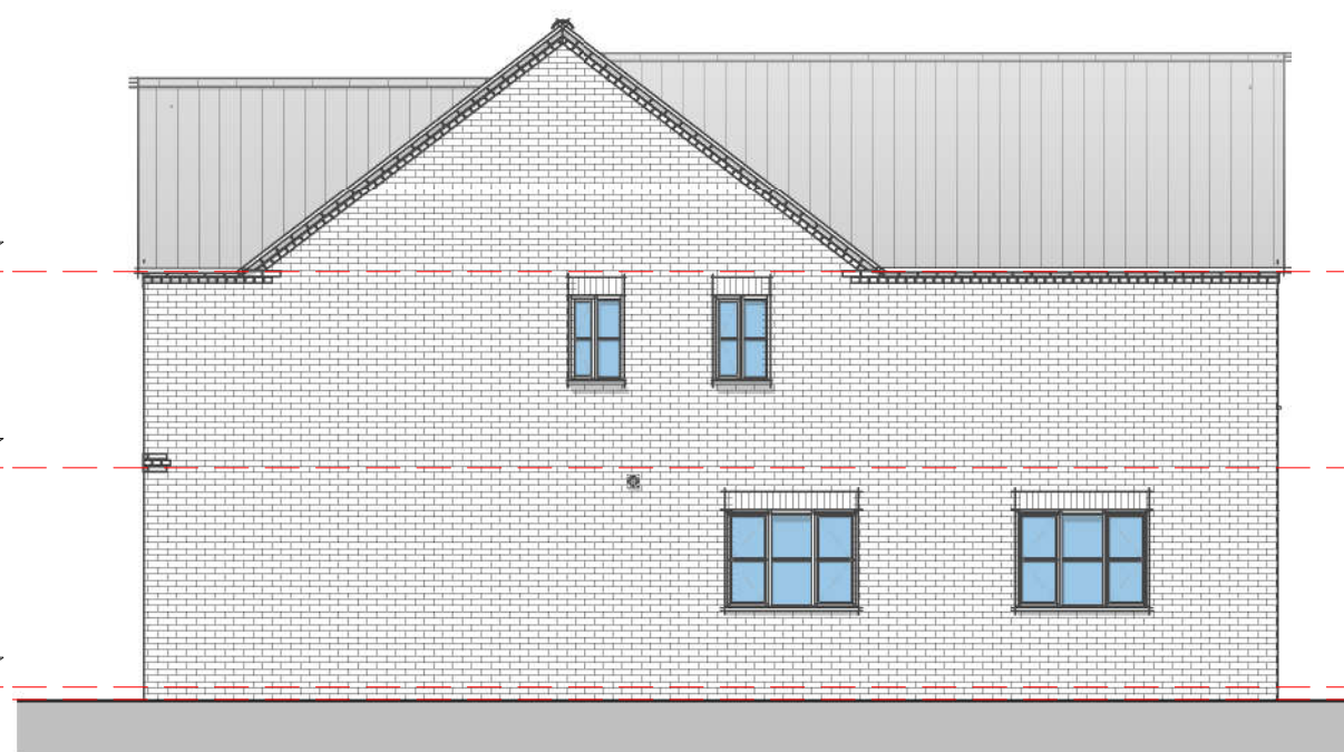
Elevation 02 - Right
