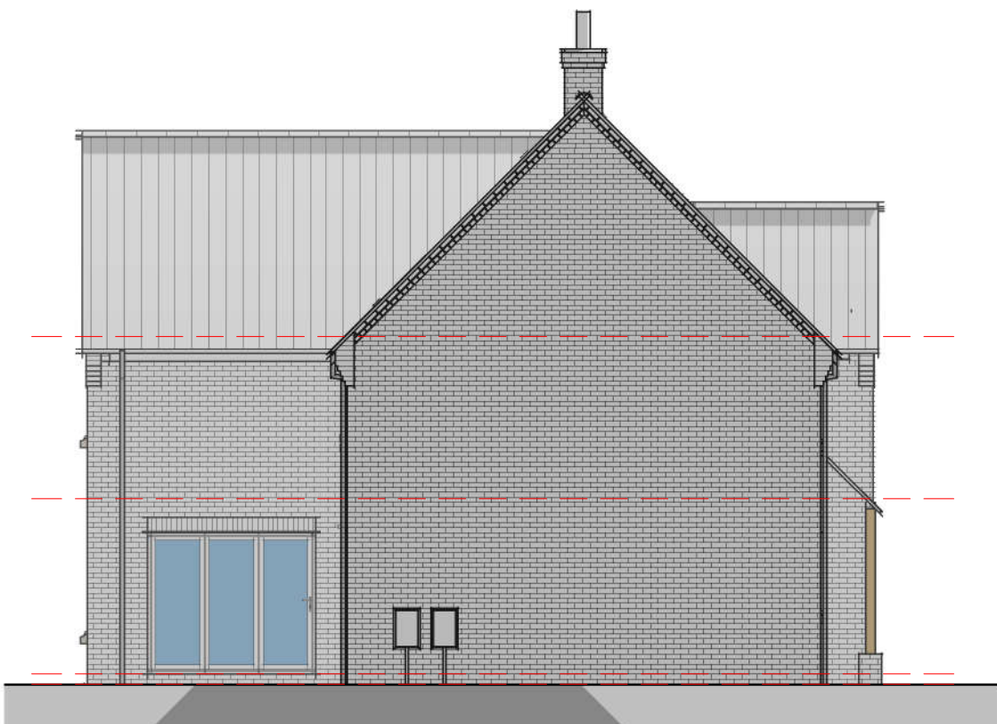
Elevation 04 - Left 1 : 100
