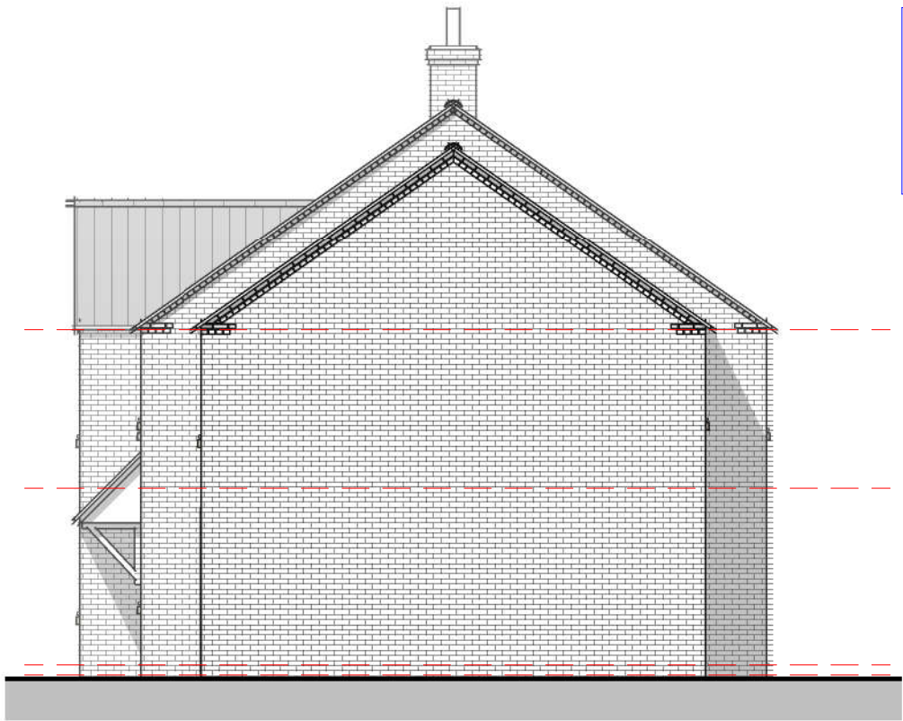
Elevation 02 - Right
