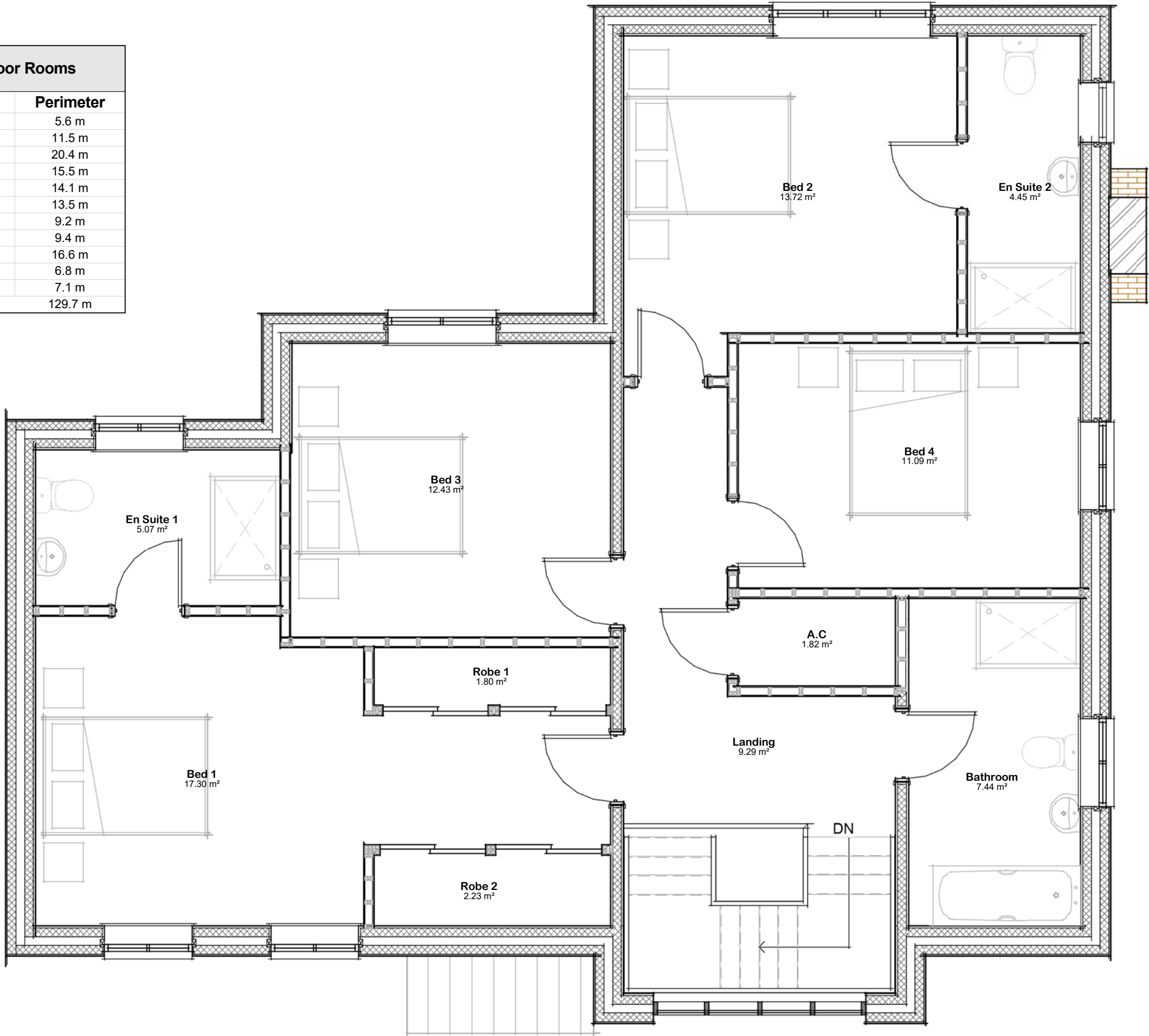
Plan 02 - First 1 : 50
