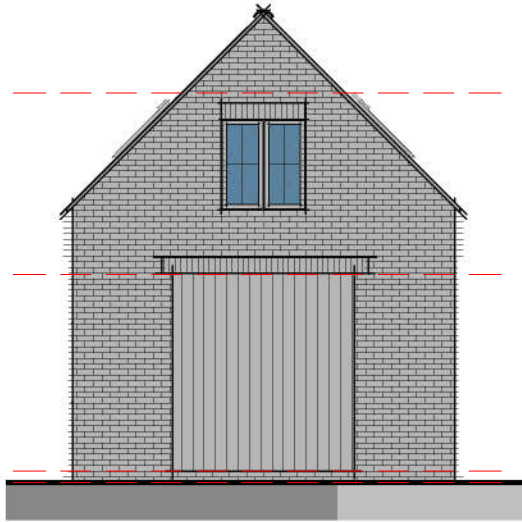
Elevation 04 - Left 1 : 100
