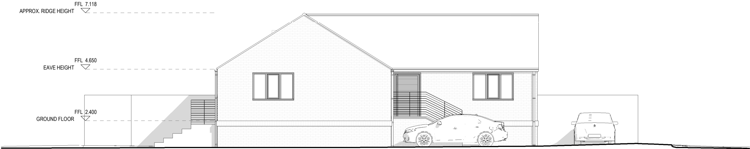
Elevation 3 1 : 100
