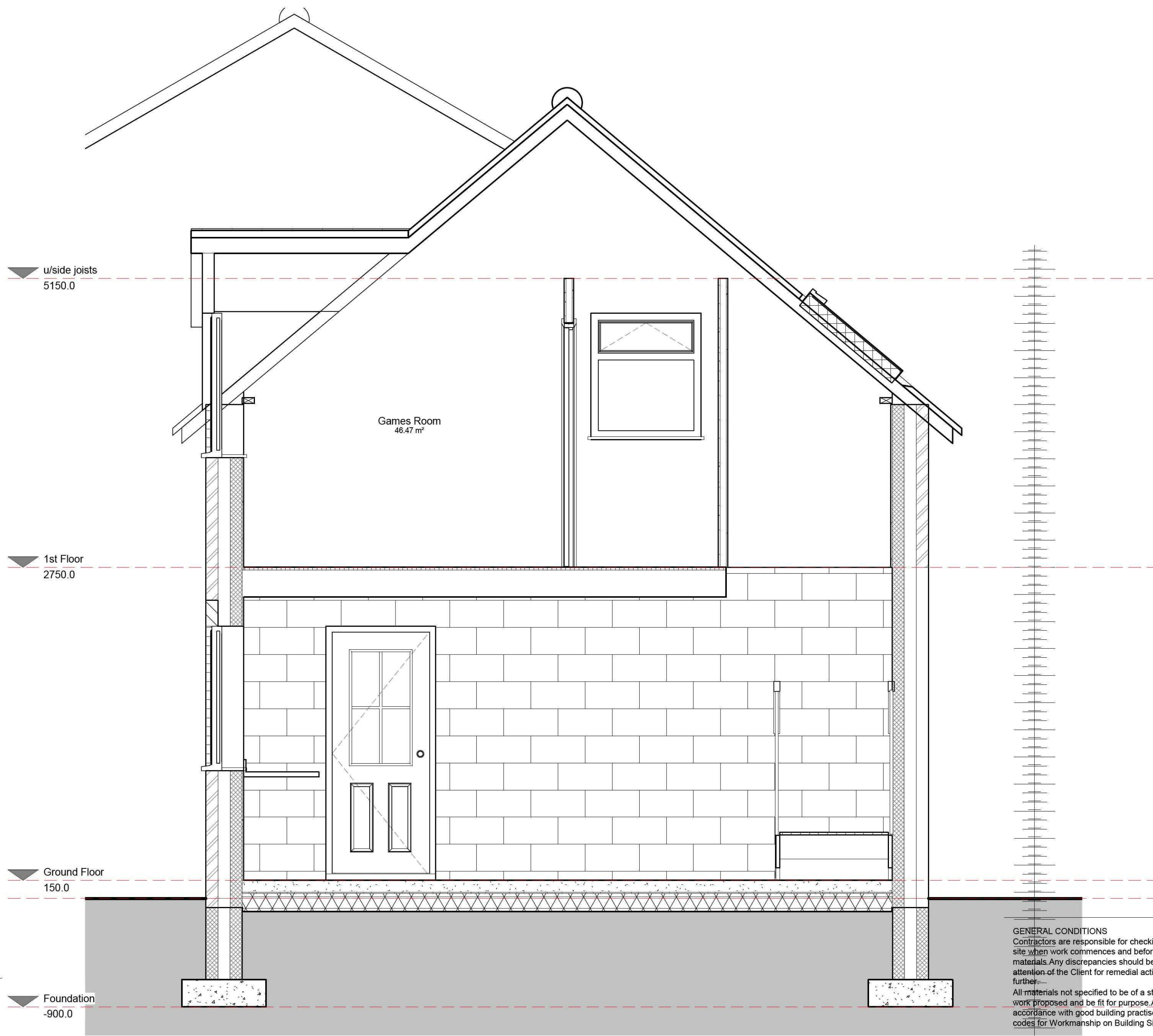
2 Garage Section 1 : 25
