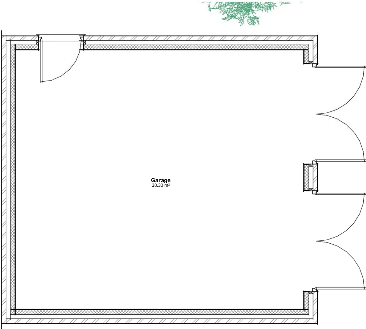
05 - Garage Plan 1 : 50
