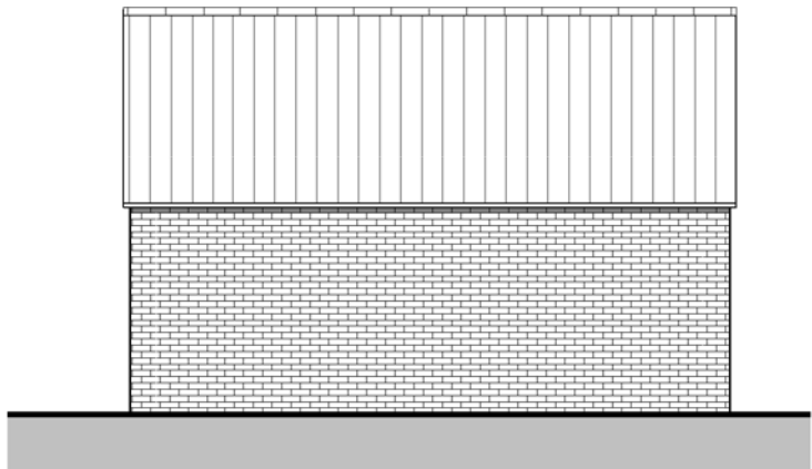
08 - Left Flank 1 : 100
