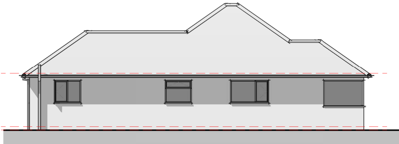
Elevation 04 - Left 1 : 100
