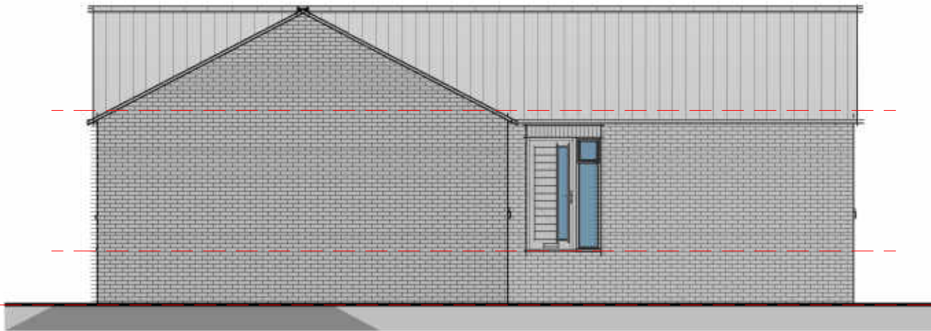
Elevation 04 - Left 1 : 100
