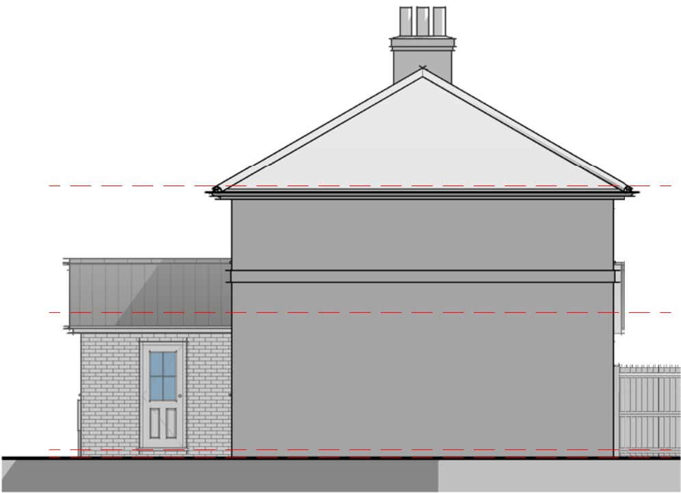
Elevation 02 - Right 1 : 100
