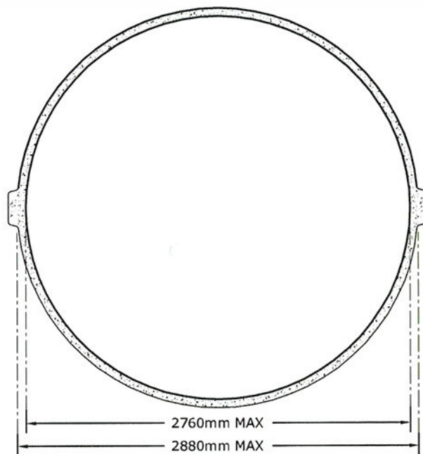
PLAN VIEW: SCALE: 1:35
