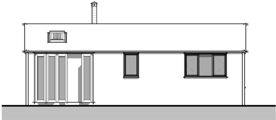
03 - Rear 1 : 100
