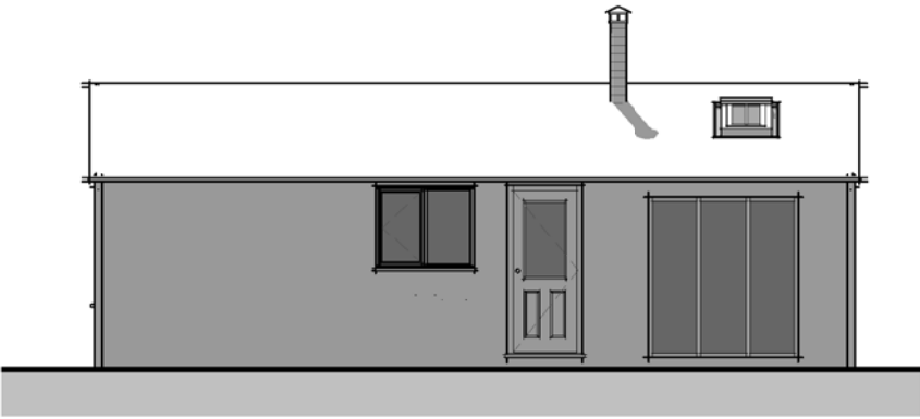
01 - Front 1 : 100
