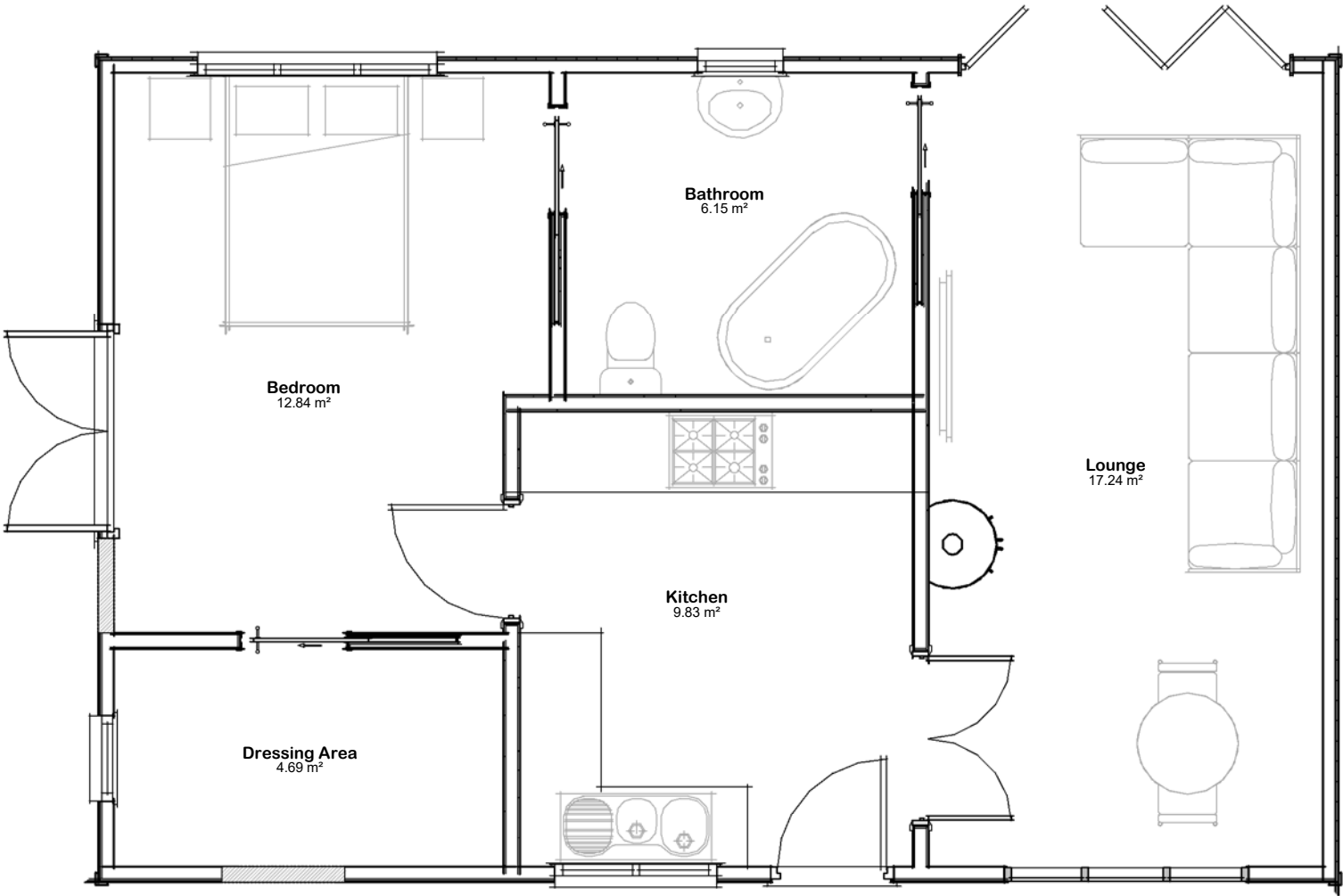
01 - Floor Plan 1 : 50
