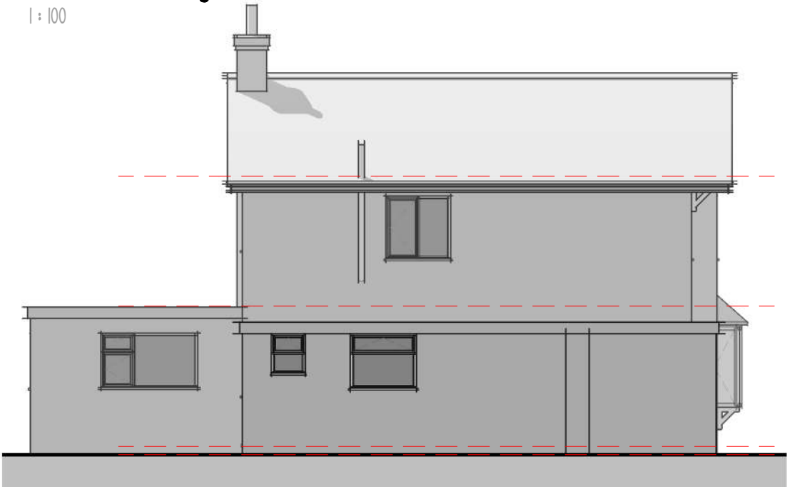
Elevation 04 - Left 1 : 100
