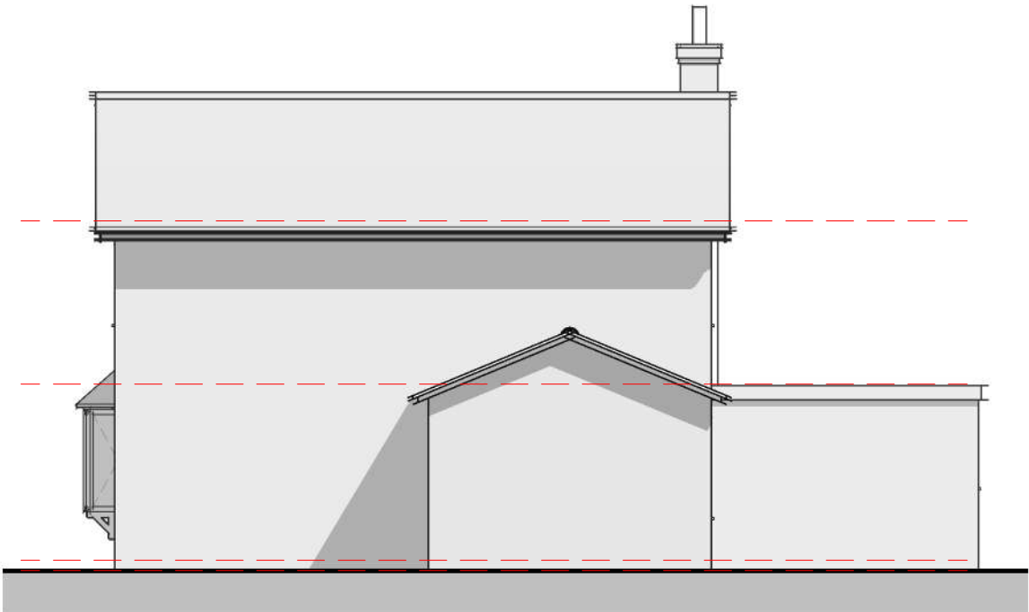
Elevation 02 - Right 1 : 100
