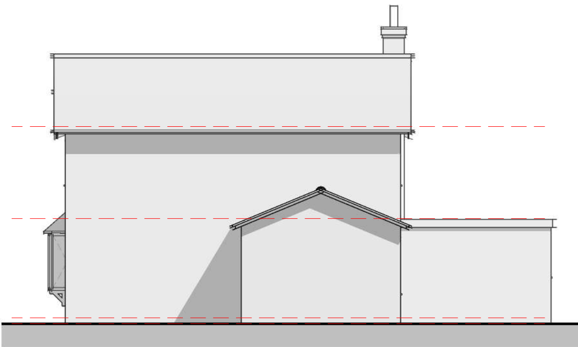
Elevation 02 - Right 1 : 100
