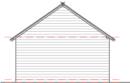
Elevation 02 - Right 1 : 100
