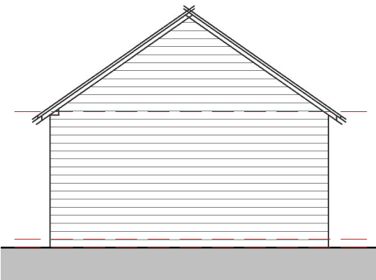
Elevation 04 - Left 1 : 100
