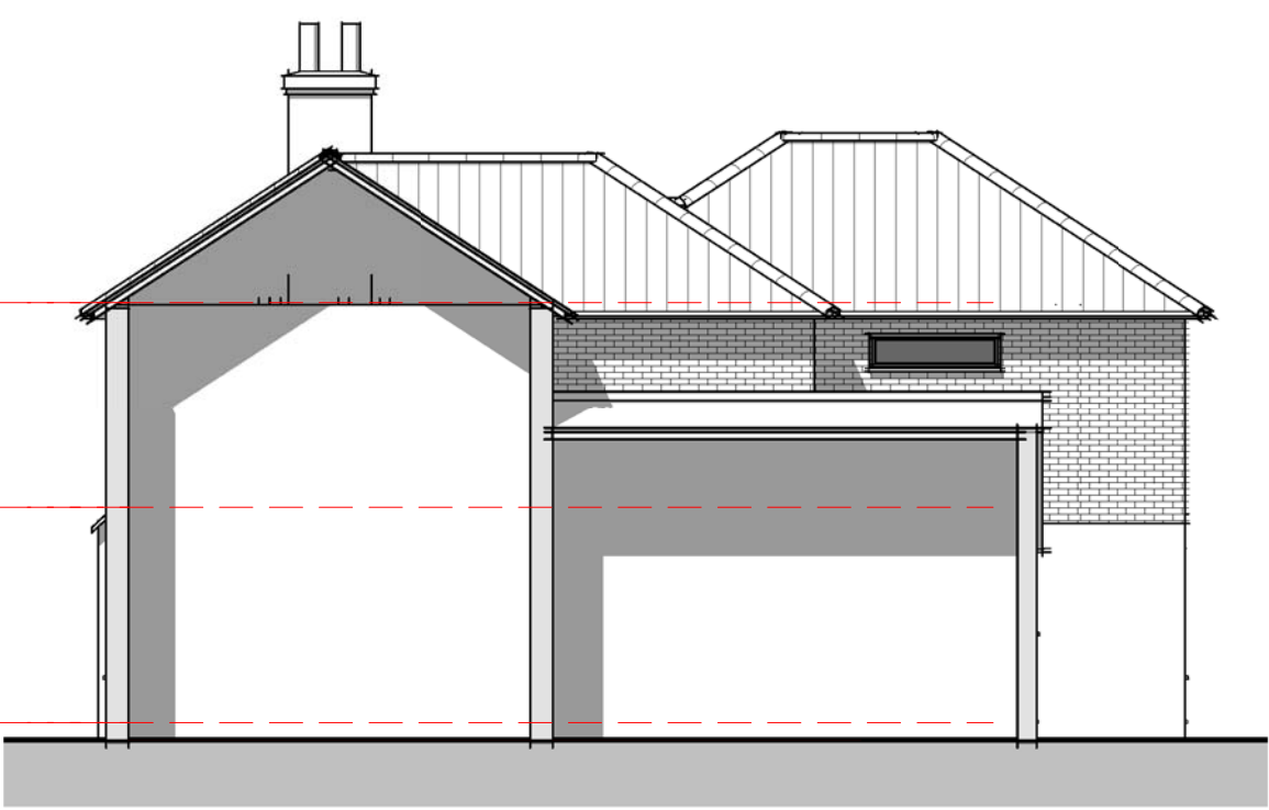
02 - Right Flank 1 : 100
