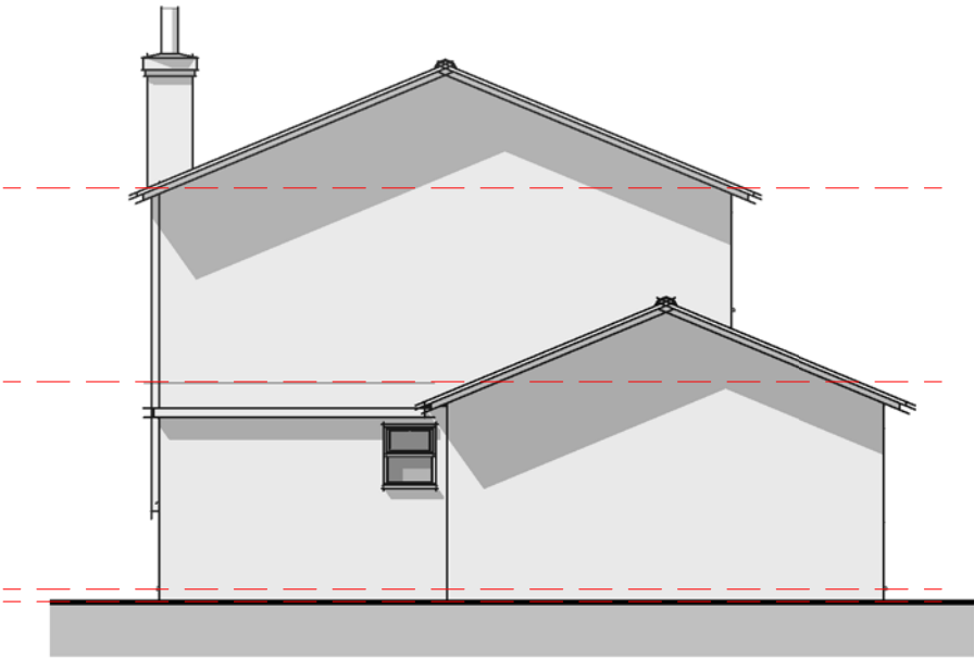
Elevation 04 - Left 1 : 100
