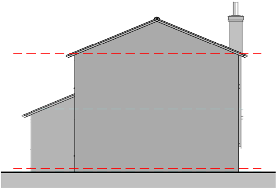
Elevation 02 - Right 1 : 100
