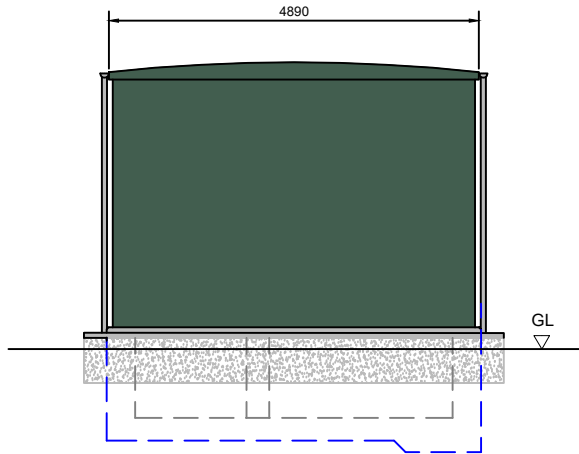
END ELEVATION
