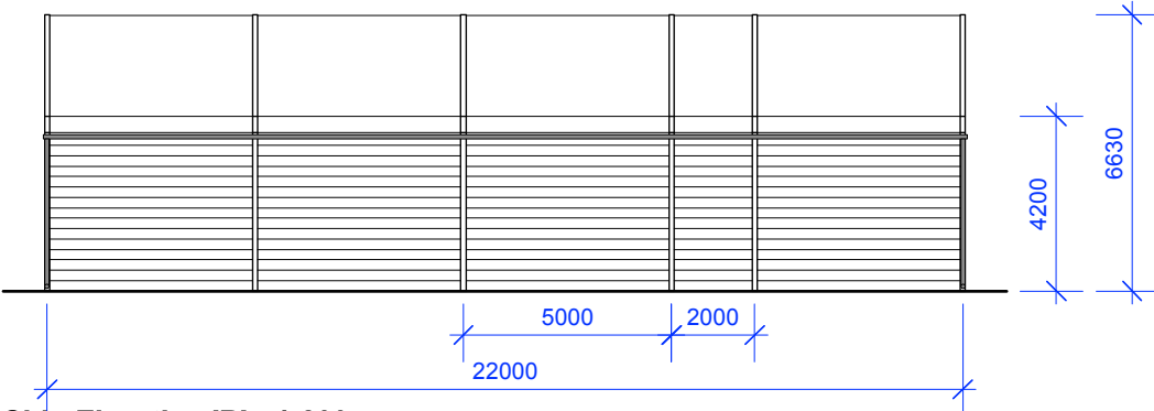
Side Elevation 'B' - 1:200
