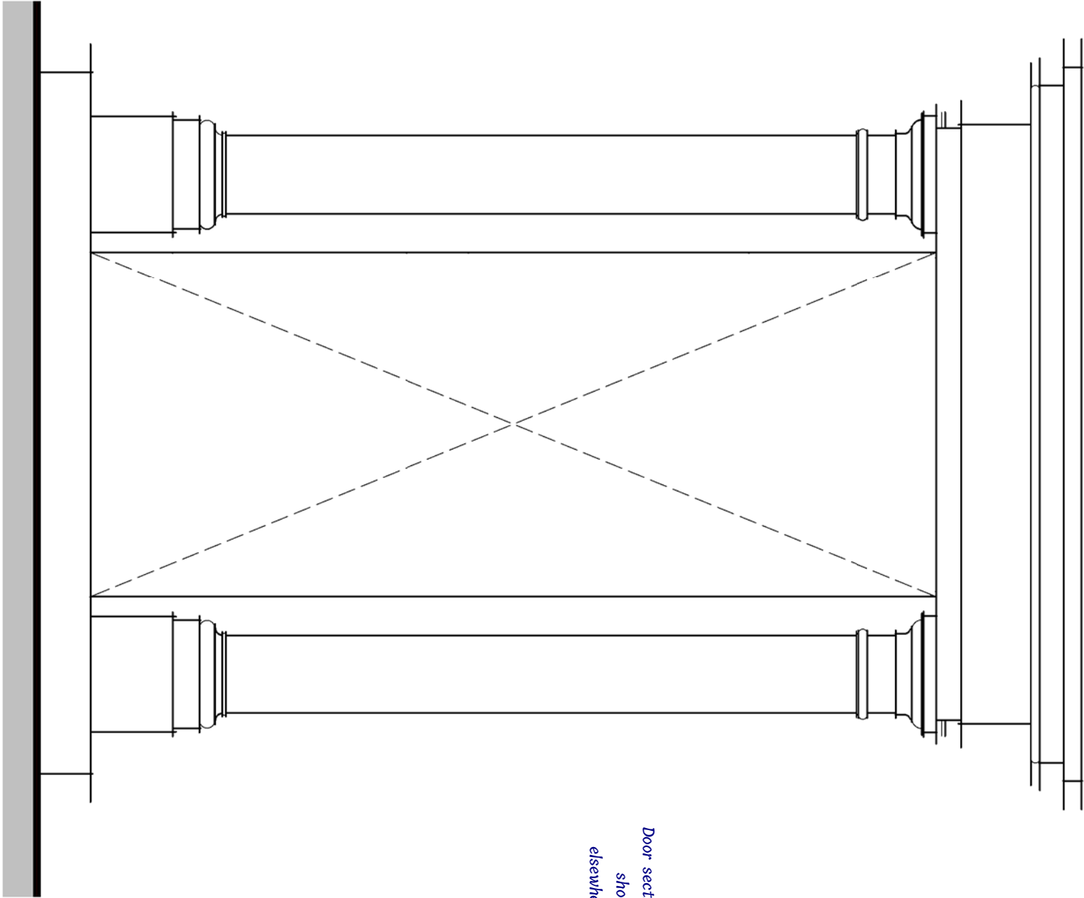
Elevation Door Surround 1 : 15
