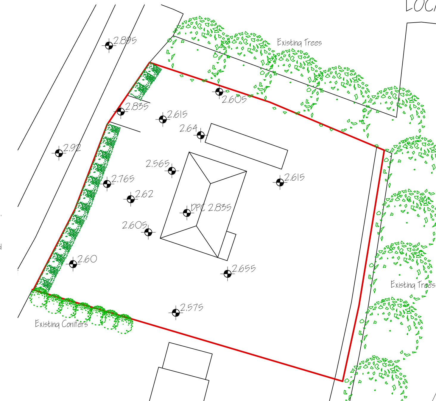
SITE PLAN - EXISTING 1:250
