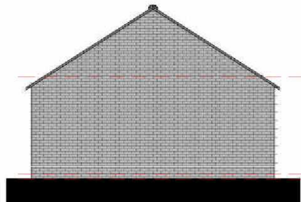
Elevation 04 - Left 1 : 100
