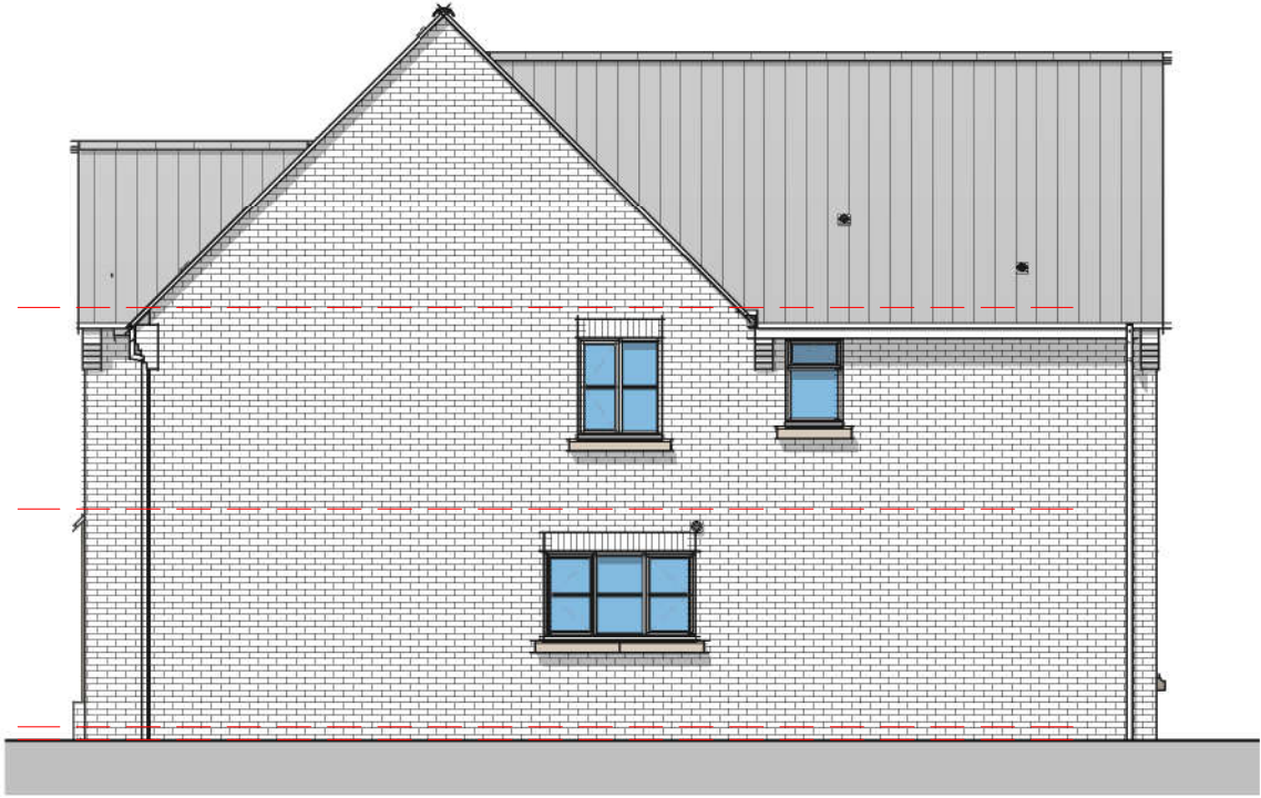
Elevation 02 - Right 1 : 100
