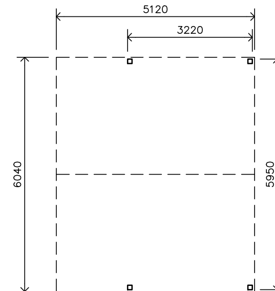
Plan 1:100
