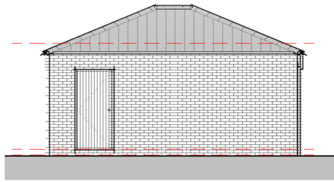
Elevation 04 - Left I : 100
