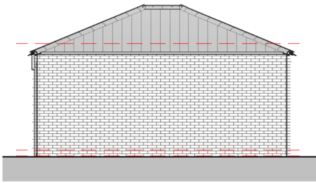
Elevation 02 - Right I : 100
