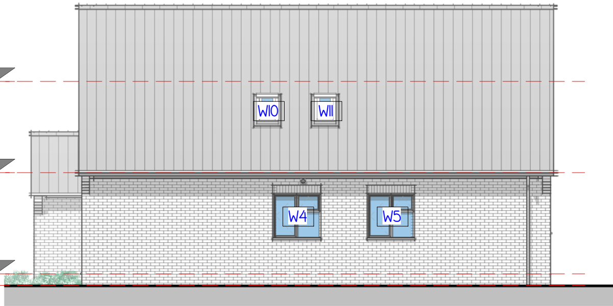
Elevation 02 - Right 1 : 100
