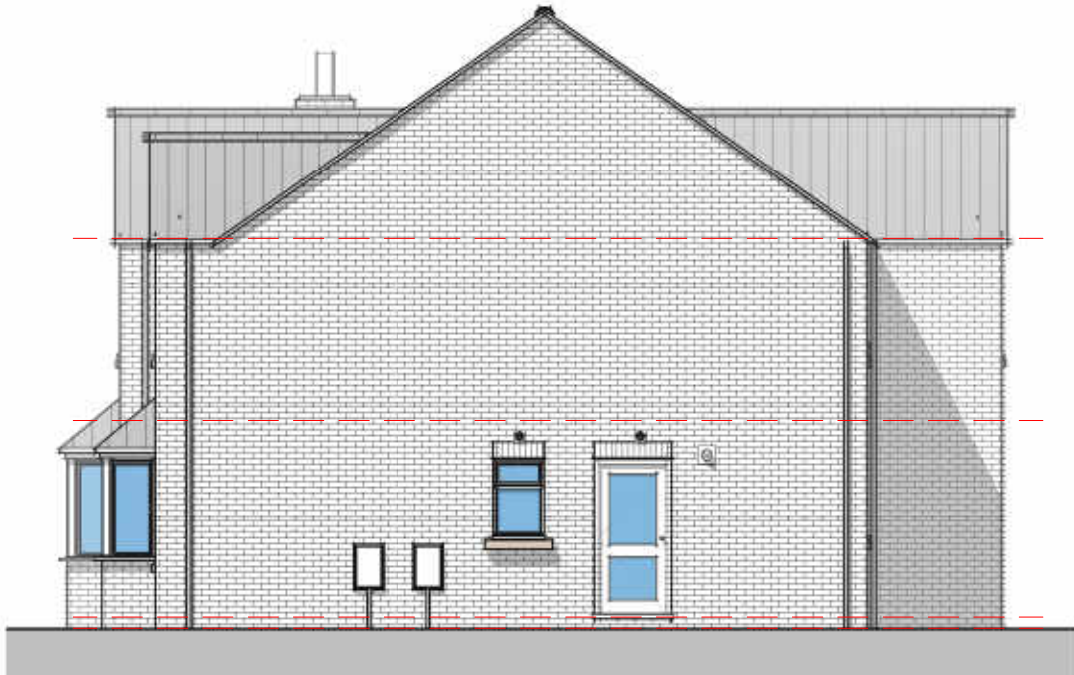
Elevation 02 - Right
