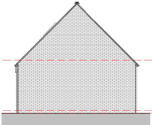
Elevation 05 - Left 1 : 100
