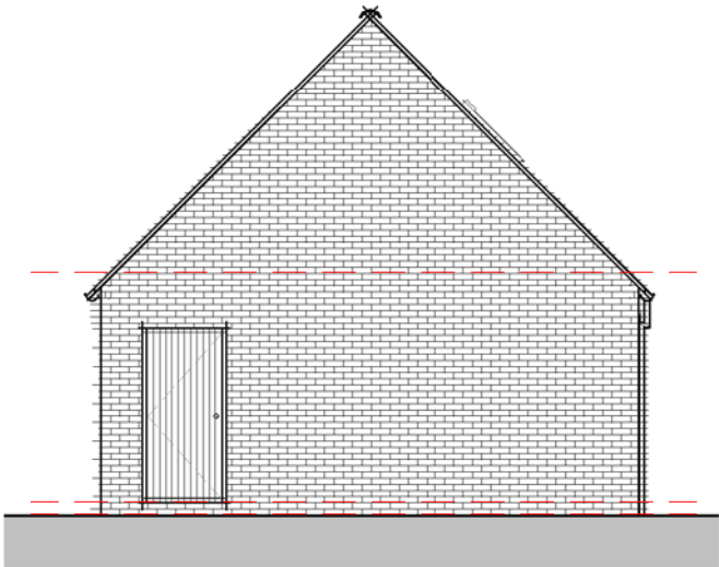
Elevation 02 - Right 1 : 100
