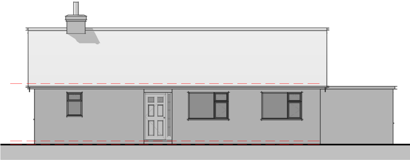
Elevation 02 - Right
