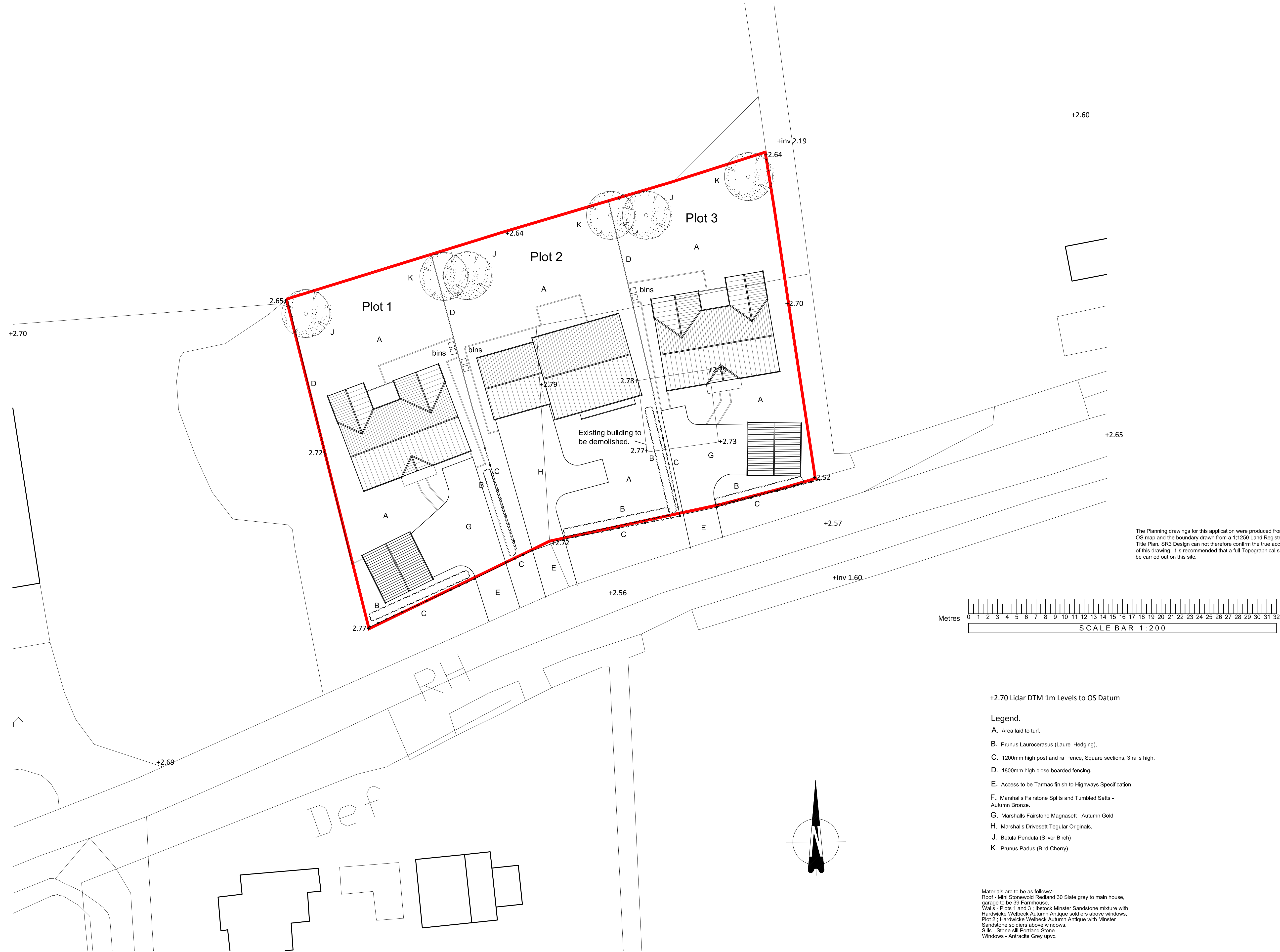
SITE PLAN 1:200
