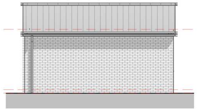
Elevation 04 - Left 1 : 100
