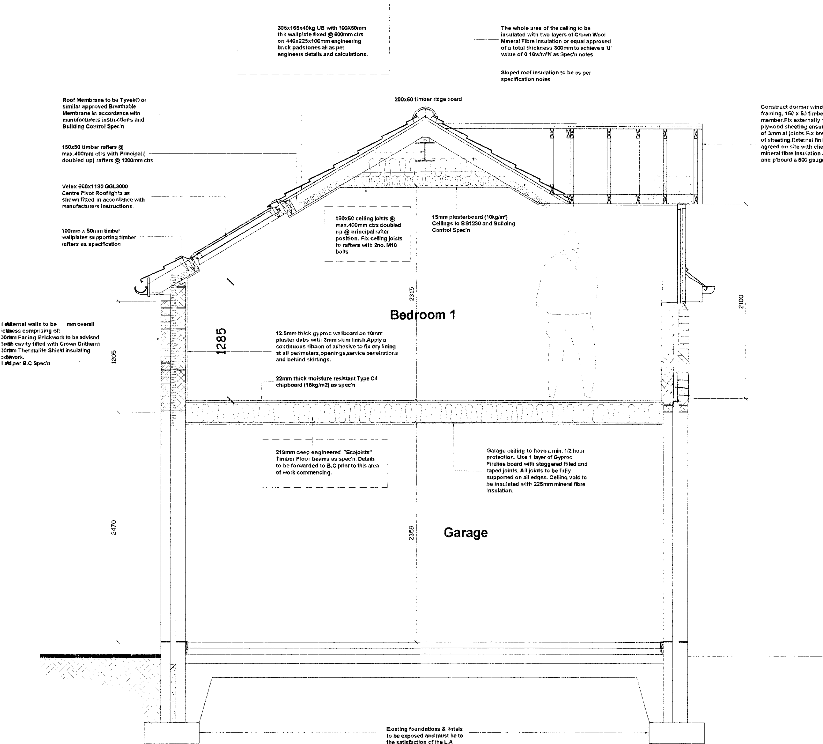
Section A-A Scale 1:25
