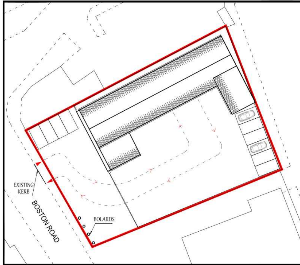
EXISTING SITE PLAN SCALE: 1/500 @A3
