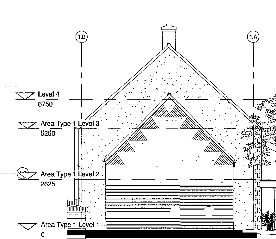
Section 1.A 1 : 100
