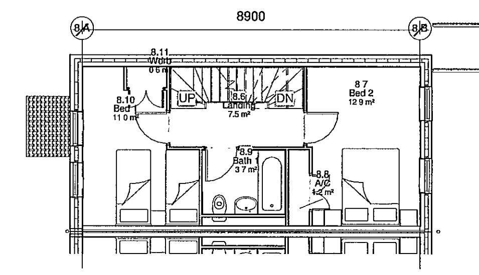
Type 8 Level 2 1 : 100
