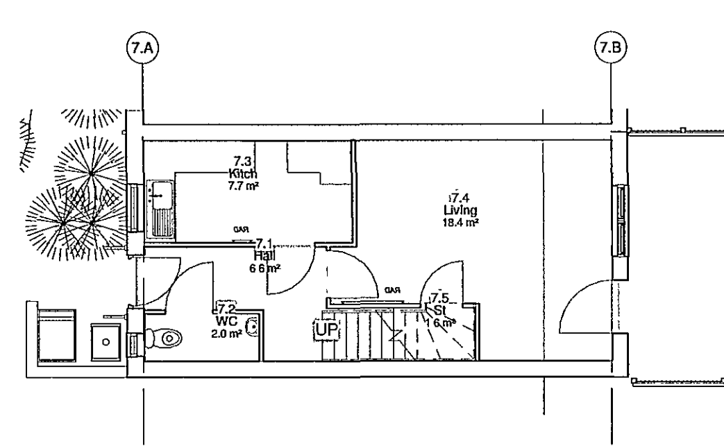
Type 6 8p 4b Rent Level 1 1 : 100
