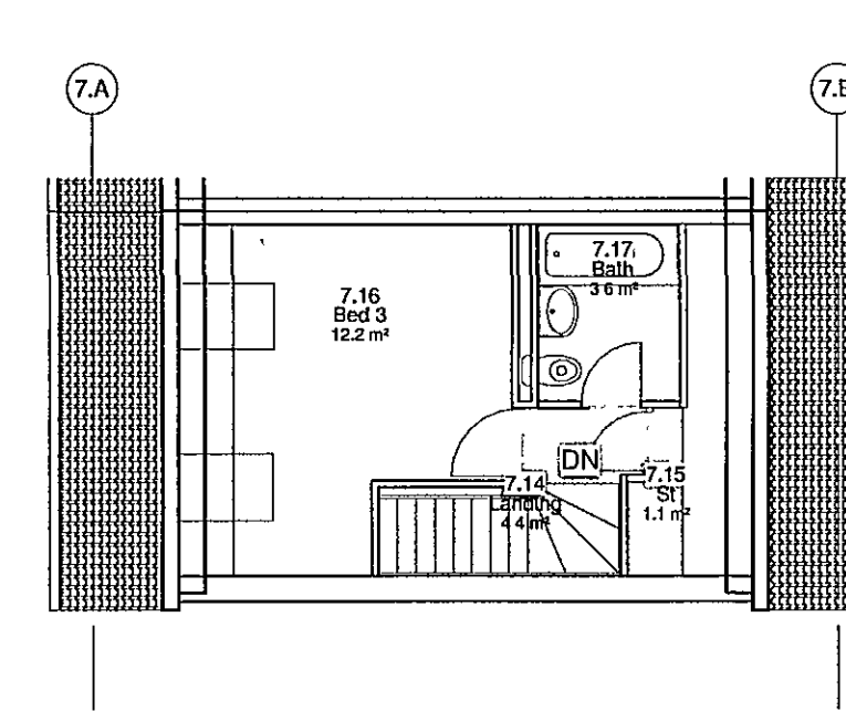
Type 6 8p 4b Rent Level 3 1 : 100
