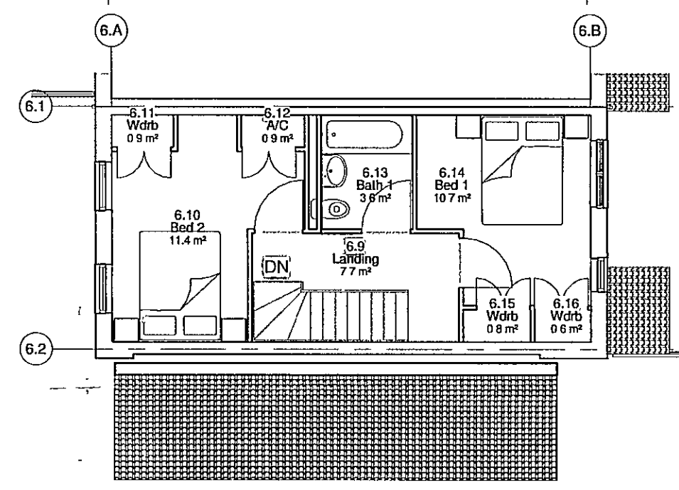
Type 6 8p 4p Rent Level 2 1 : 100
