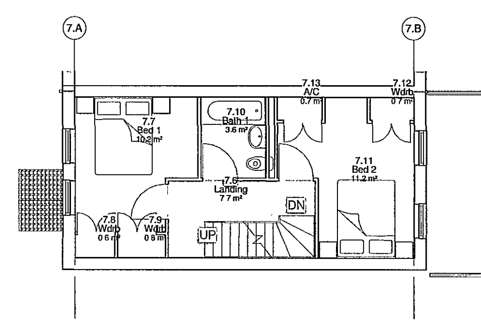
Type 7 Level 2 1 : 100
