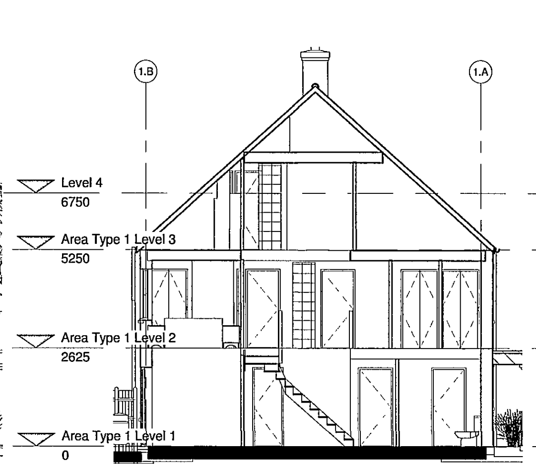
Section 1.B 1 : 100
