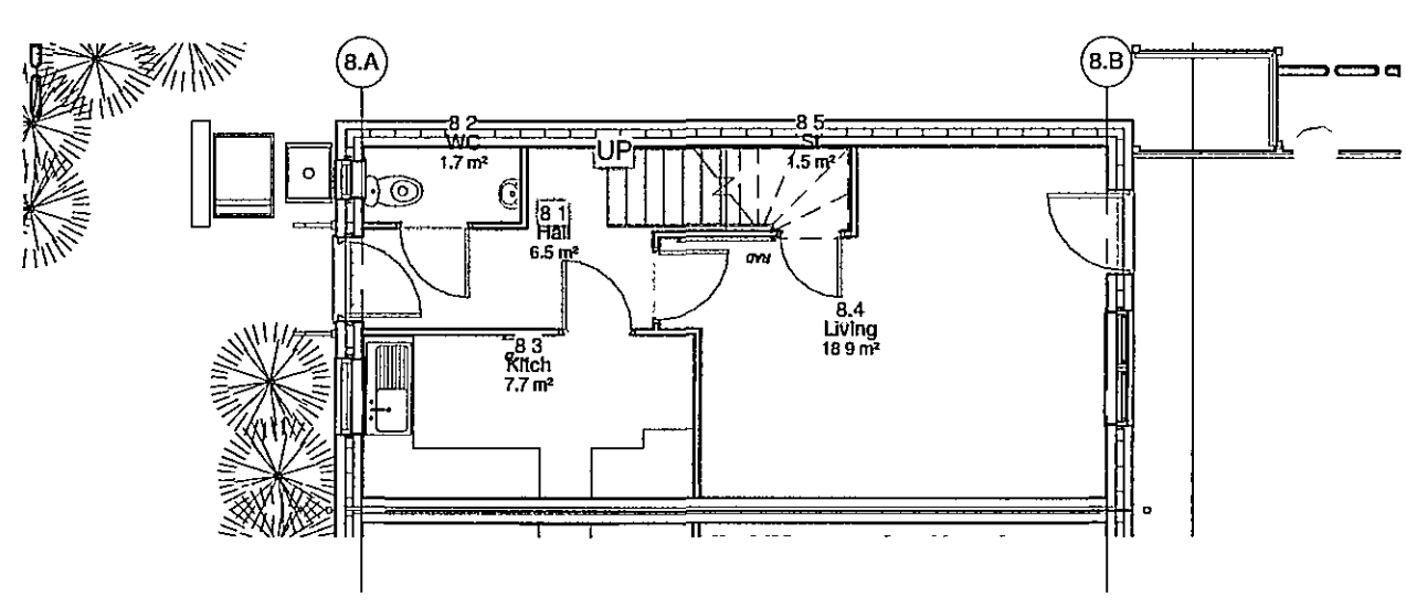
Type 8 Level 1 1 : 100
