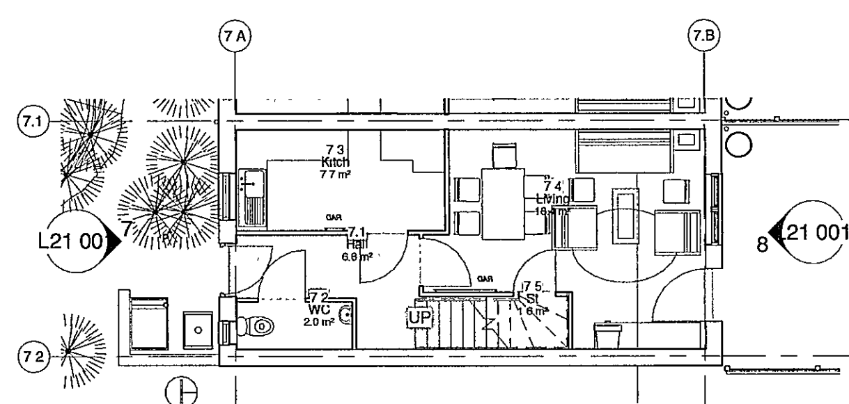
Type 6 8p 4b Rent Level 1 1 : 100
