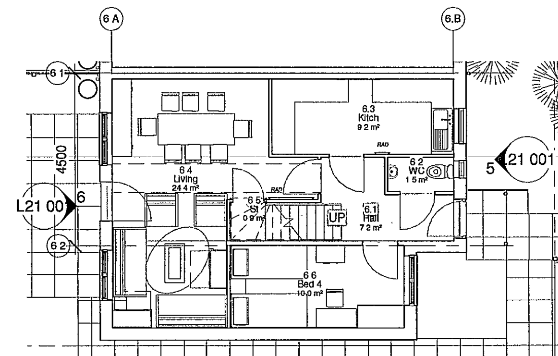
Type 6 8p 4b Rent Level 1 1 : 100
