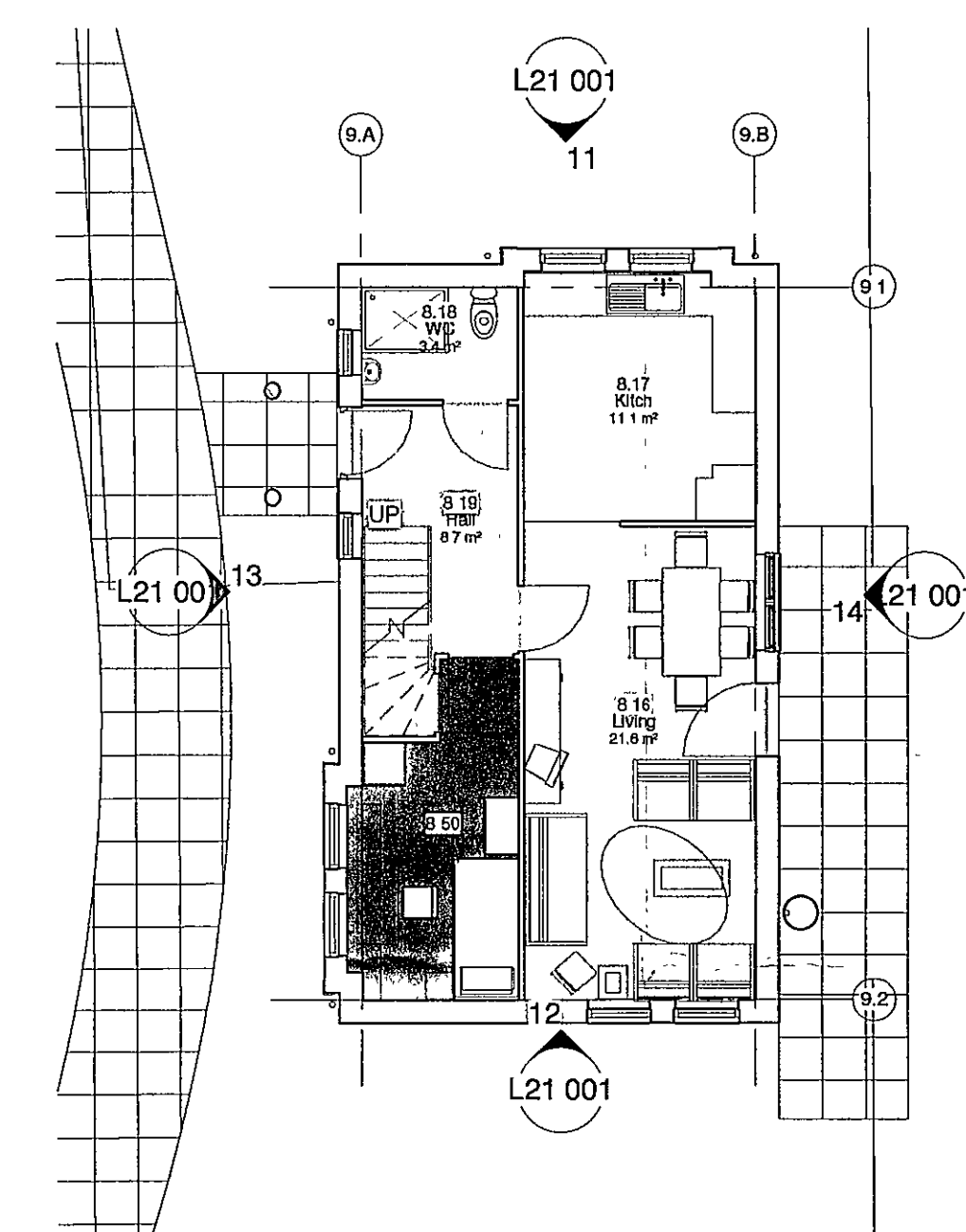
Type 9 Level 1 1 : 100
