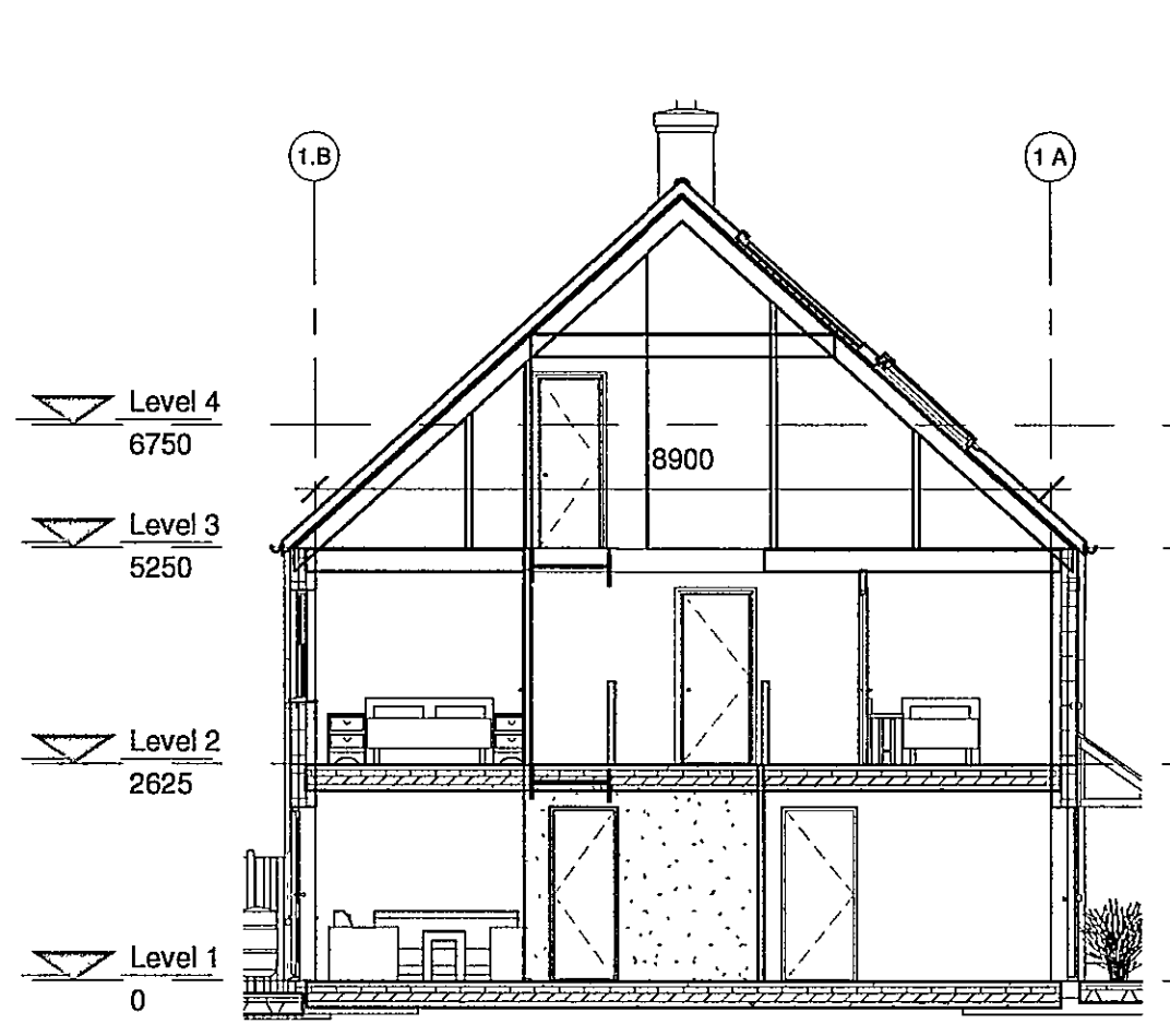
Section 1.B 1 : 100
