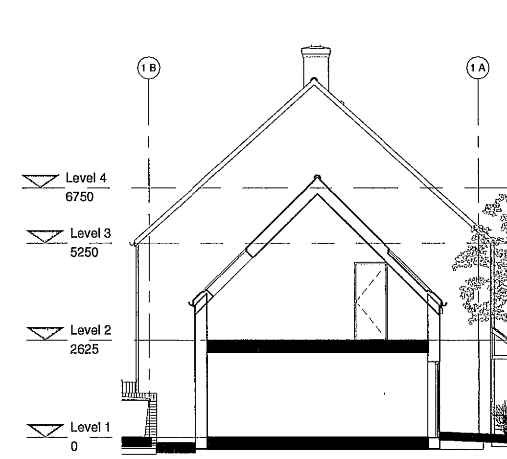
Section 1.A 1 : 100
