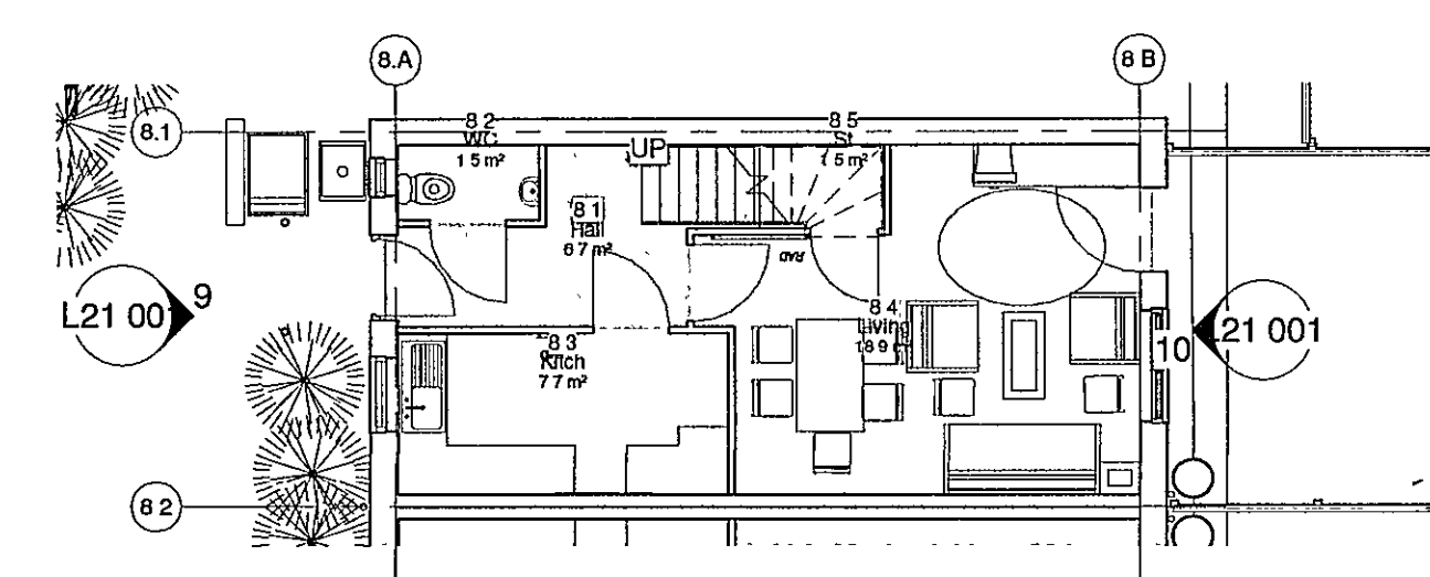
Type 8 Level 1 1 : 100
