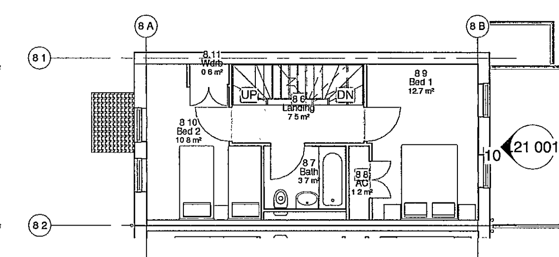
Type 8 Level 2 1 : 100
