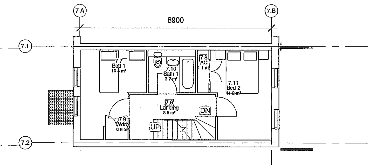
Type 7 Level 2 1 : 100
