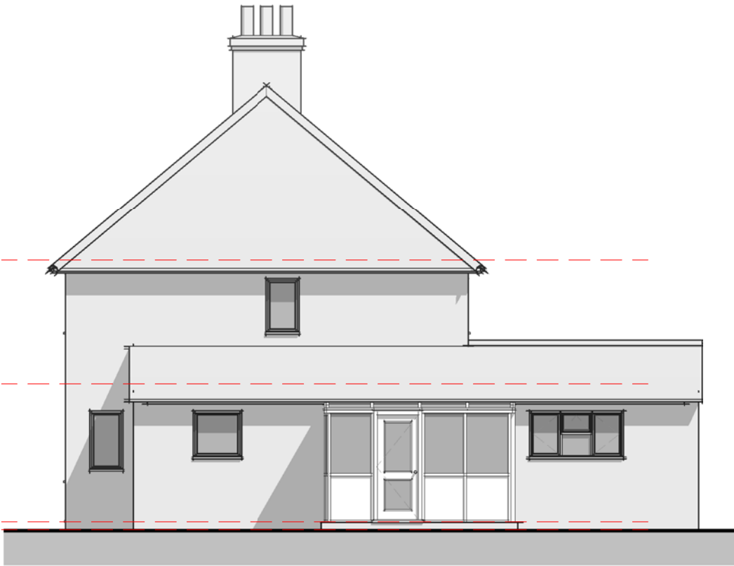
Elevation 02 - Right 1 : 100
