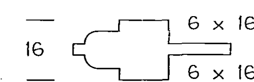
GLAZING BAR
