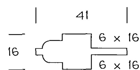
GLAZING BAR
