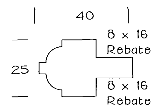
GLAZING BAR
