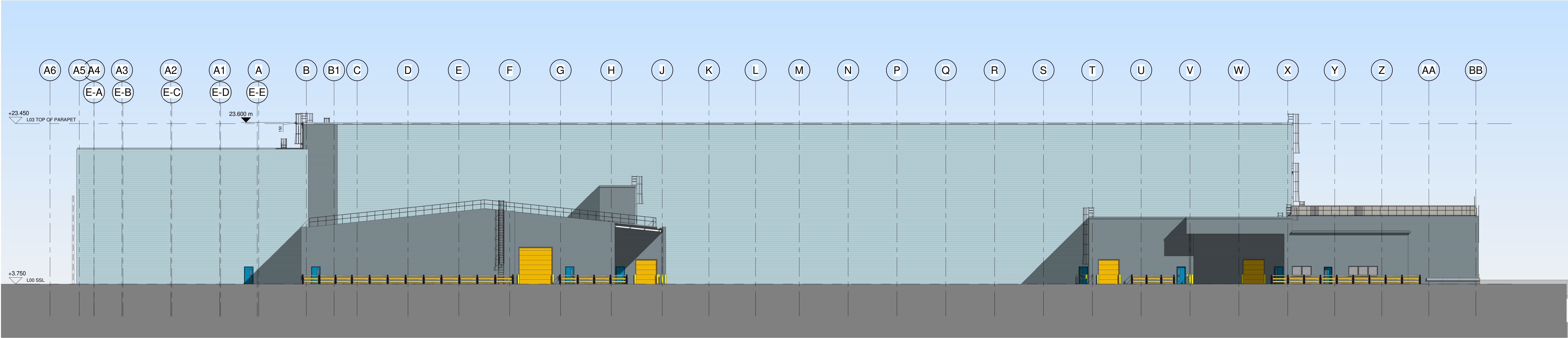
Elevation 1 1 : 200
