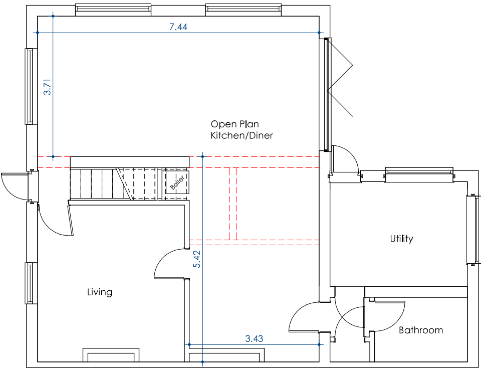
1 L0 FFL Pr 1 : 50
