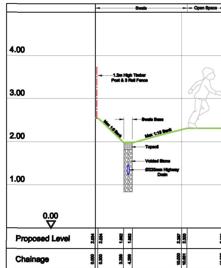
Section A-A: Scale - Horiz 1:50 Vert 1:250
