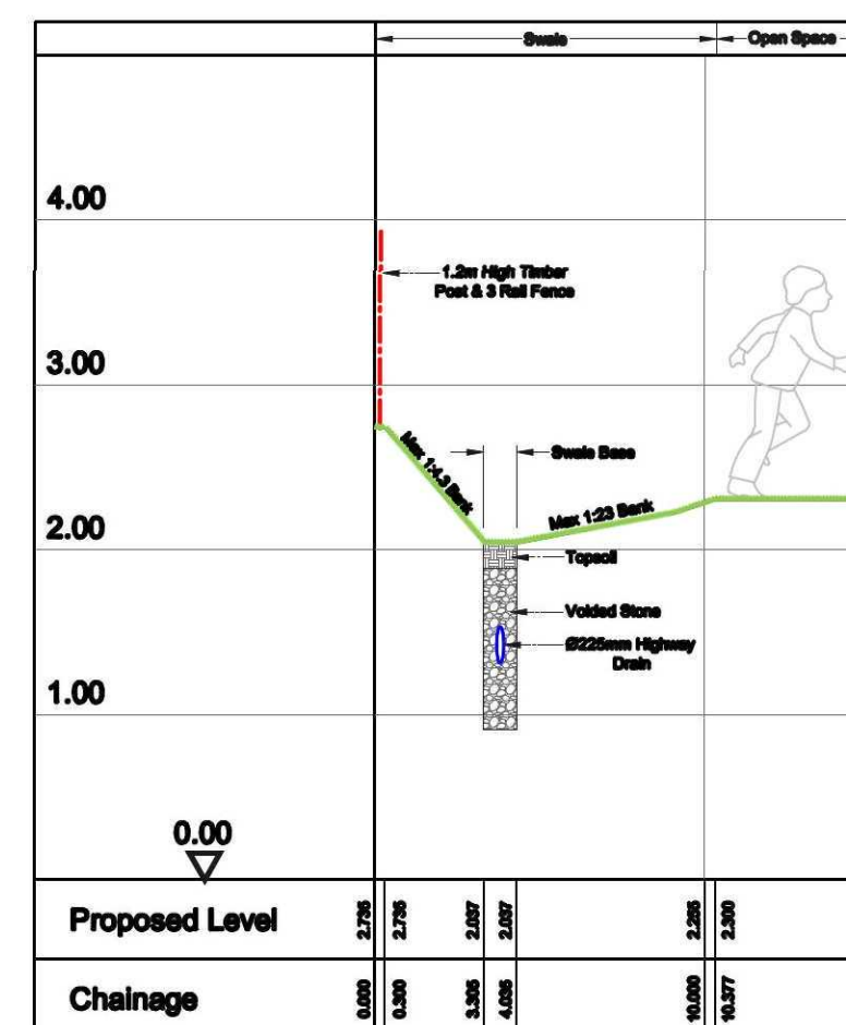
Section G-G: Scale - Horiz 1:50 Vert 1:250
