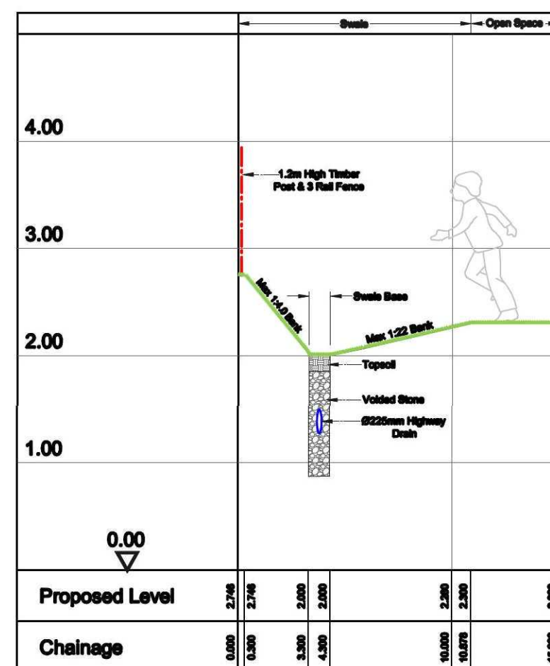
Section D-D: Scale - Horiz 1:50 Vert 1:250
