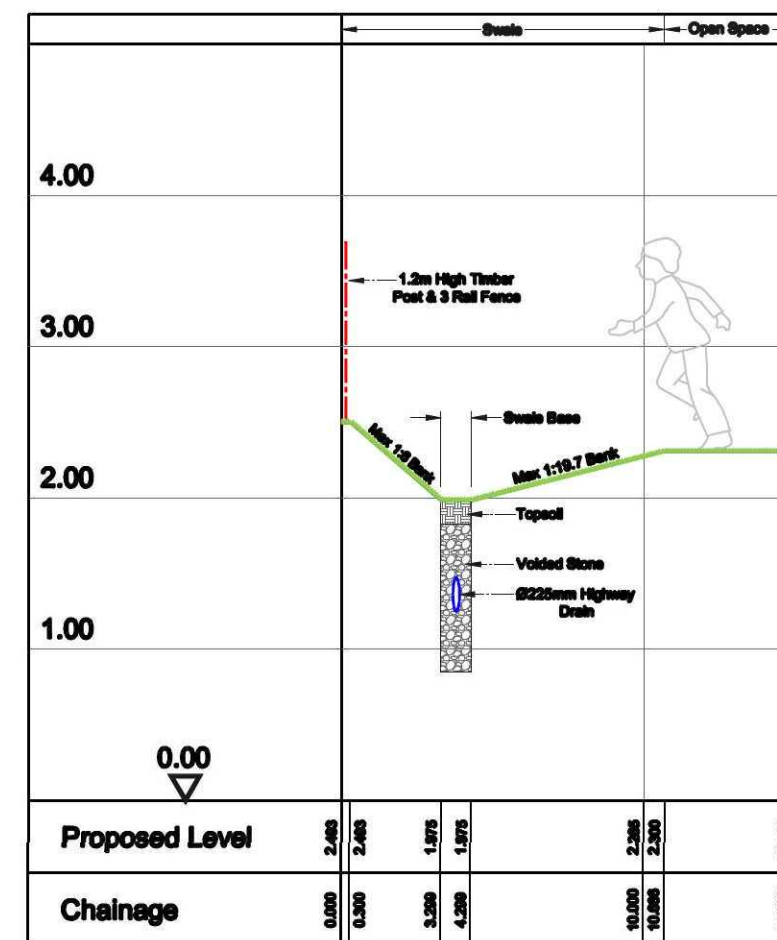
Section B-B: Scale - Horiz 1:50 Vert 1:250
