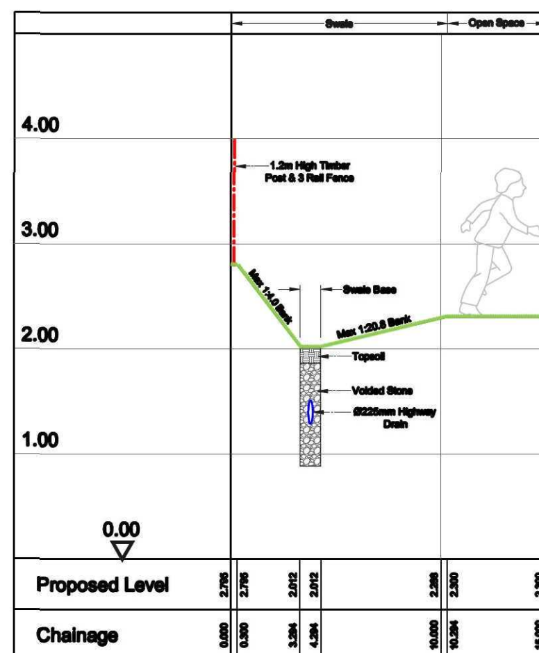
Section E-E: Scale - Horiz 1:50 Vert 1:250
