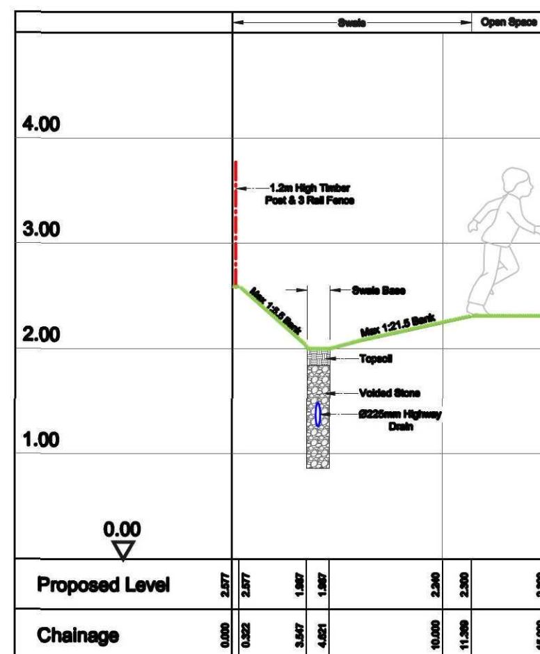
Section C-C: Scale - Horiz 1:50 Vert 1:250
