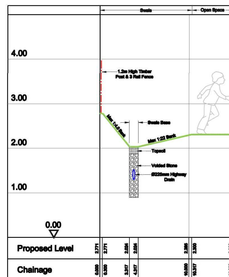
Section F-F: Scale - Horiz 1:50 Vert 1:250
