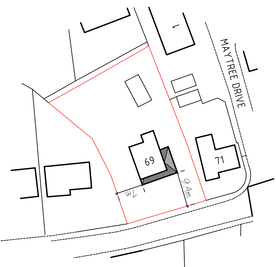
SITE PLAN. 1/500.
