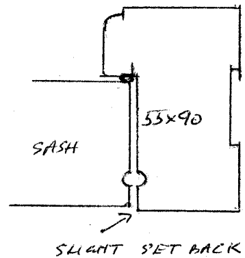
JAMB DETAIL
