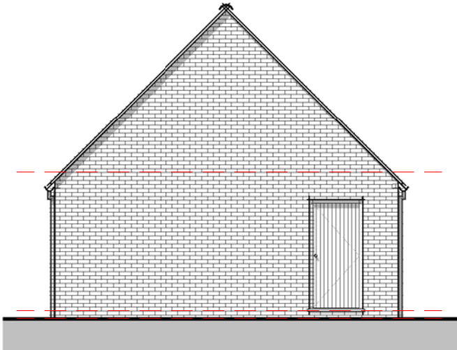
Elevation 02 - Right 1 : 100
