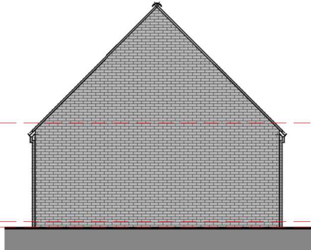
Elevation 04 - Left 1 : 100
