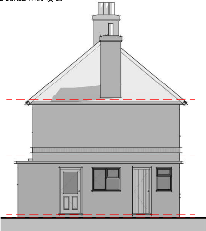
Elevation 02 - Right
