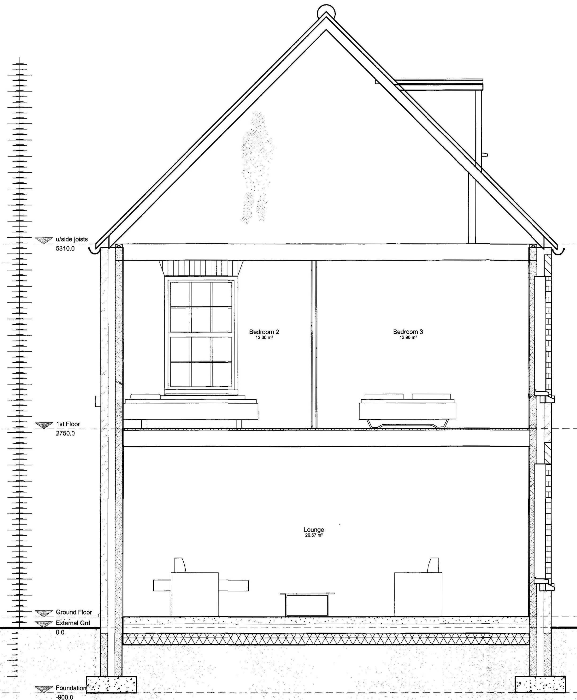
2 Main Section 1 : 25
