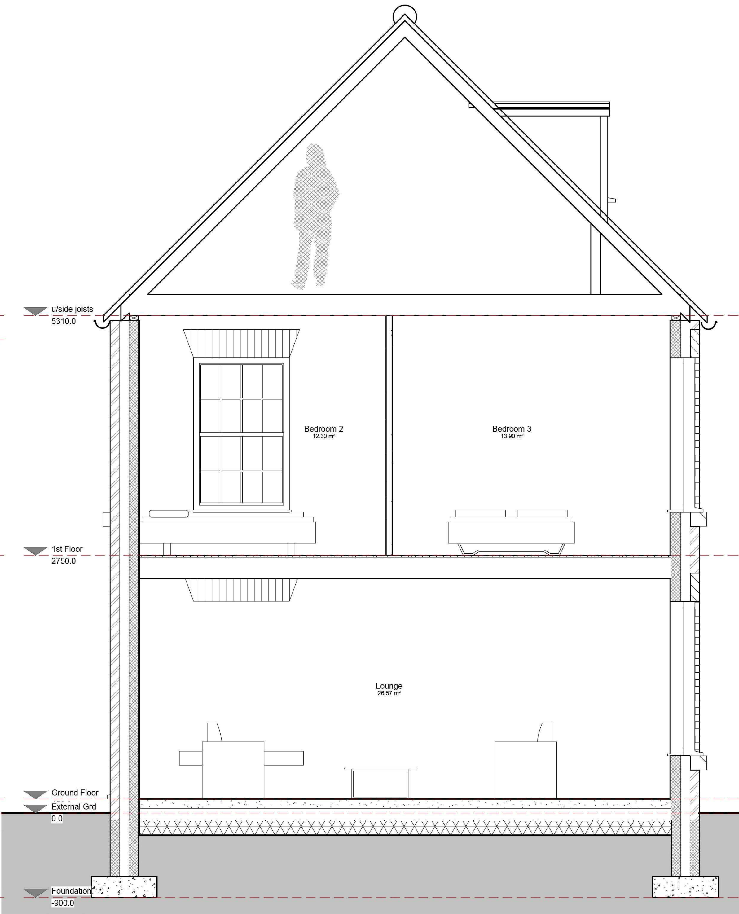
2 Main Section 1 : 25
