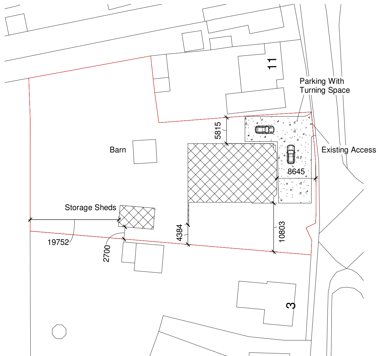
Block Plan 1 : 500
