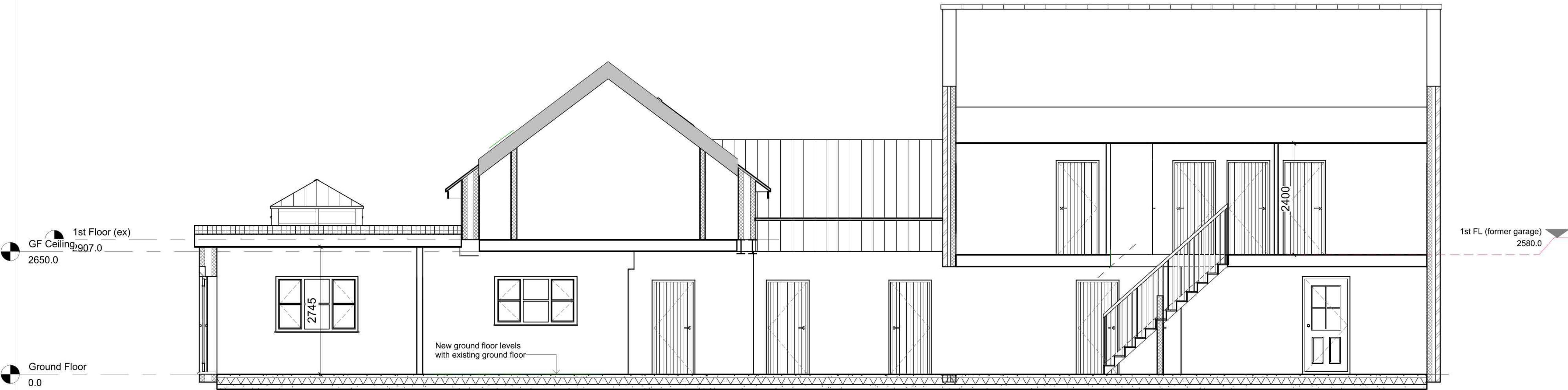
Section A-A 1 : 50
